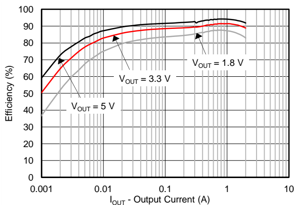
Tps562200 效率
