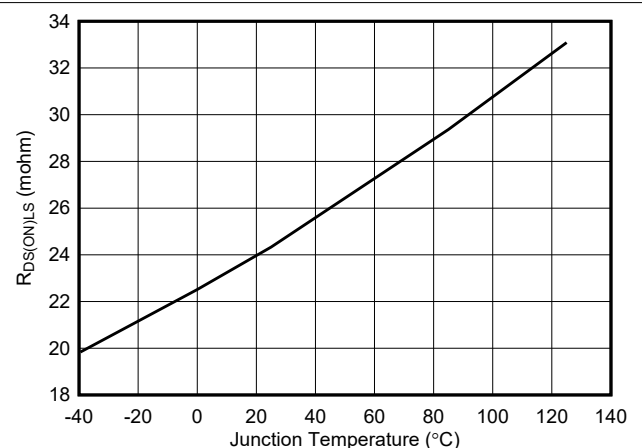
图 6-4. Low-Side R_{DS(ON)}
