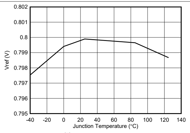
图 6-6. V_{REF} Voltage
