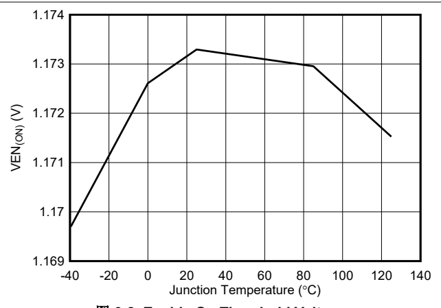
图 6-2. Enable On Threshold Voltage
