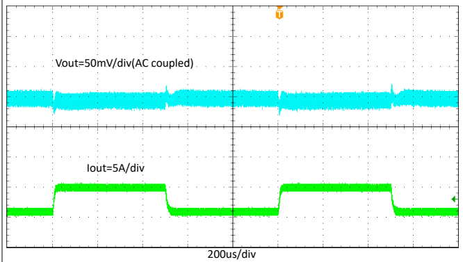
图 8-11. TPS565242 瞬态响应, 0.5A 至 4.5A, 负载阶跃为 2.5A/μs
