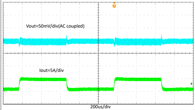
图 8-13. TPS565247 瞬态响应, 0.5A 至 4.5A, 负载阶跃为 2.5A/μs
