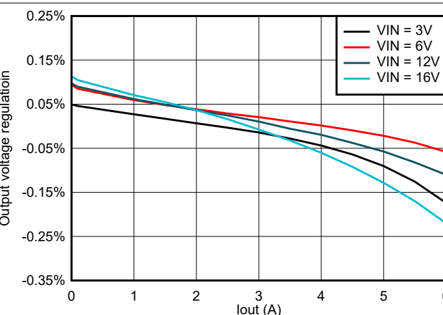
图 8-5. TPS566247 负载调整率与负载间的关系
