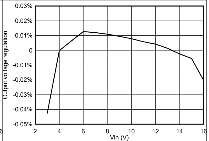
图 8-7. TPS566247 线性调整率与 V_{IN} 间的关系 (6A 负载)
