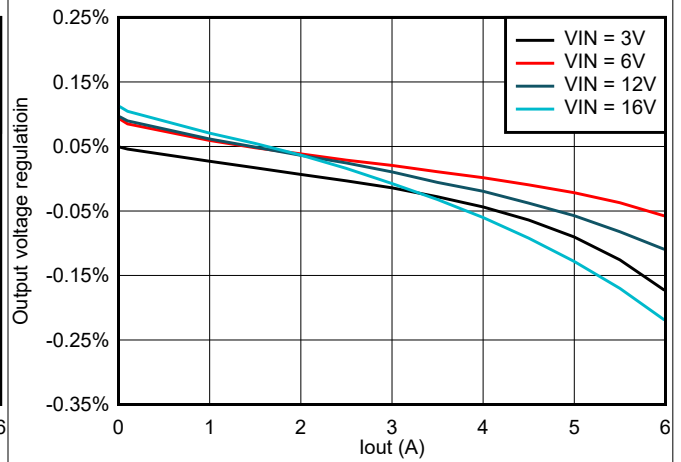
图 8-5. TPS566247 负载调整率与负载间的关系
