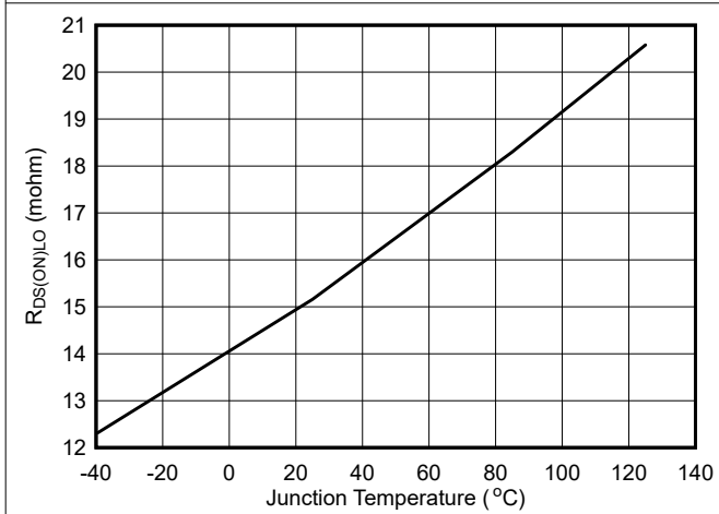
图 6-5. 低侧 R_{DS(ON)}
