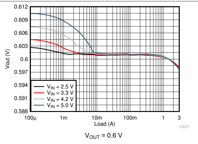
图 9-4. Load Regulation
