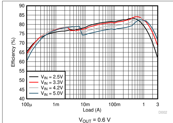
图 9-3. Efficiency
