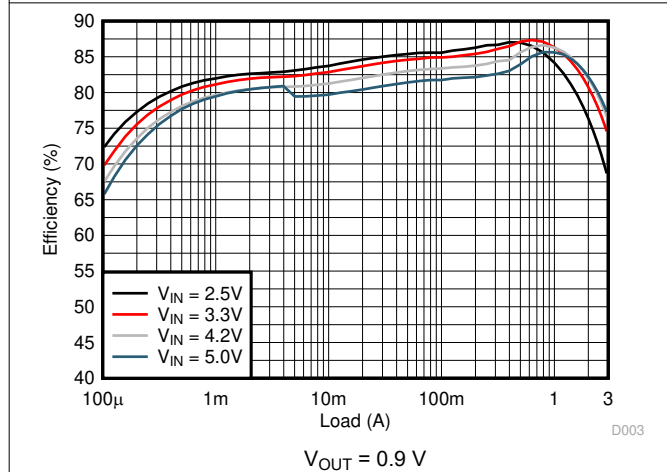
图 9-7. Efficiency
