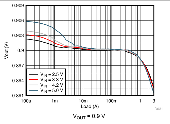
图 9-8. Load Regulation
