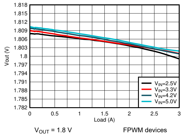
图 9-18. Load Regulation
