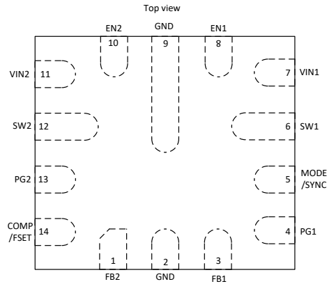
图 6-1. 14-Pin VQFN-HR RQR Package
