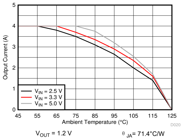
图 9-29. Thermal Derating
