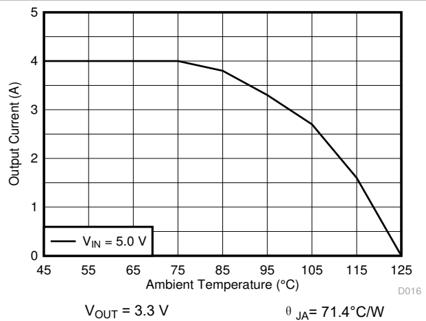
图 9-32. Thermal Derating
