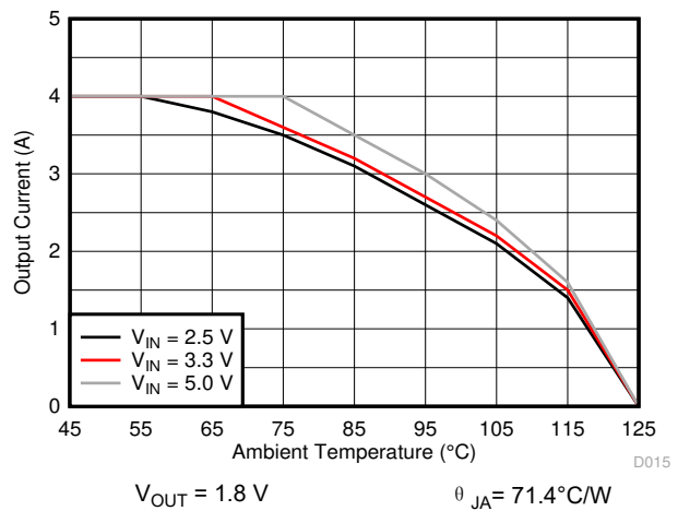
图 9-30. Thermal Derating
