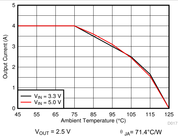
图 9-31. Thermal Derating
