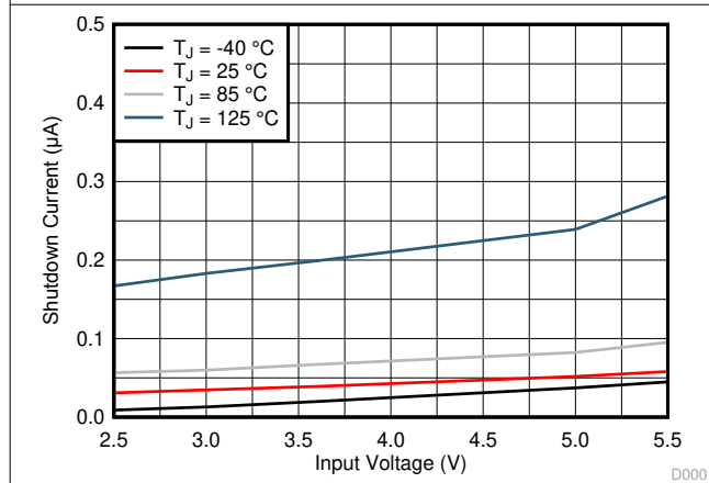
图 7-3. Shutdown Current
