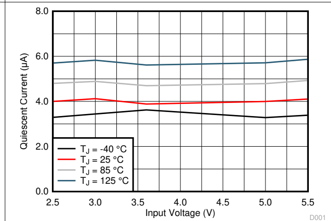
图 7-4. Quiescent Current
