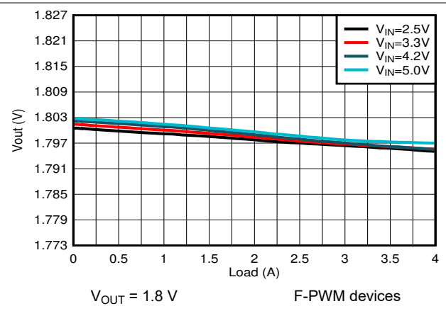
图 9-14. Load Regulation
