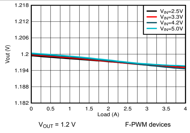
图 9-10. Load Regulation
