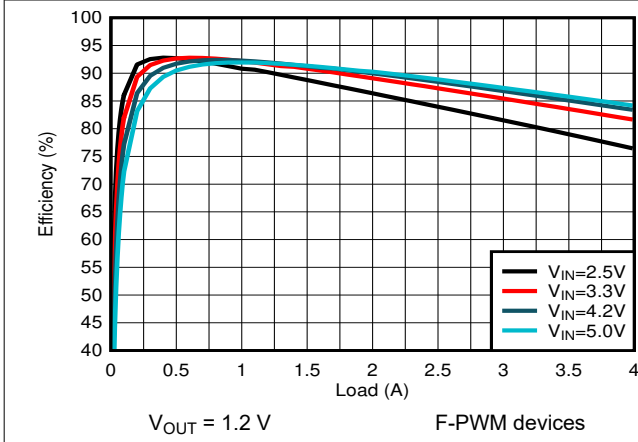
图 9-9. PWM Efficiency
