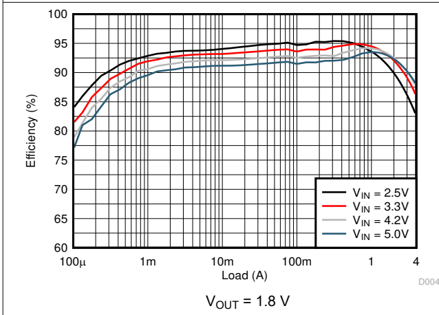
图 9-11. Efficiency
