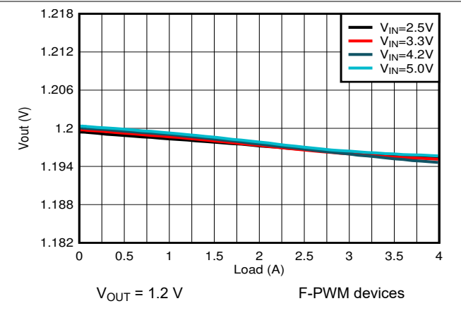
图 9-10. Load Regulation
