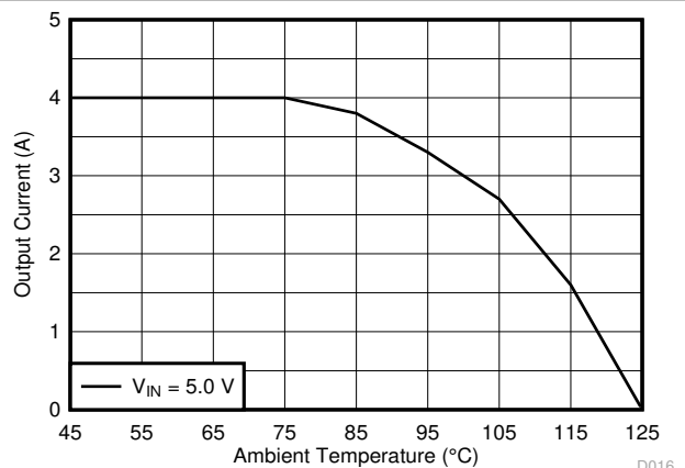
图 9-30. Thermal Derating
