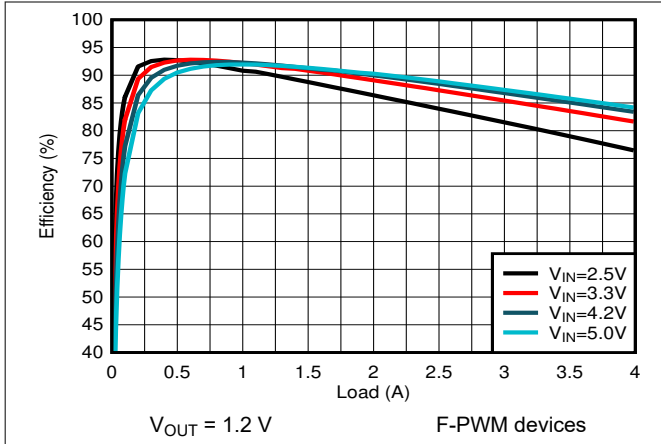
图 9-9. PWM Efficiency
