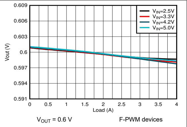
图 9-6. Load Regulation
