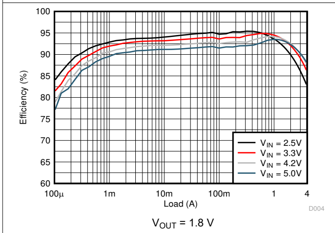
图 9-11. Efficiency
