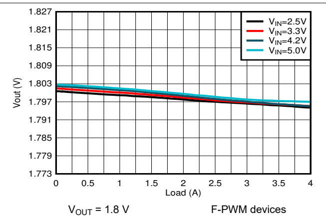
图 9-14. Load Regulation
