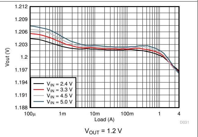
图 9-8. Load Regulation
