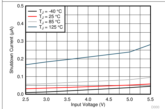
图 7-3. Shutdown Current
