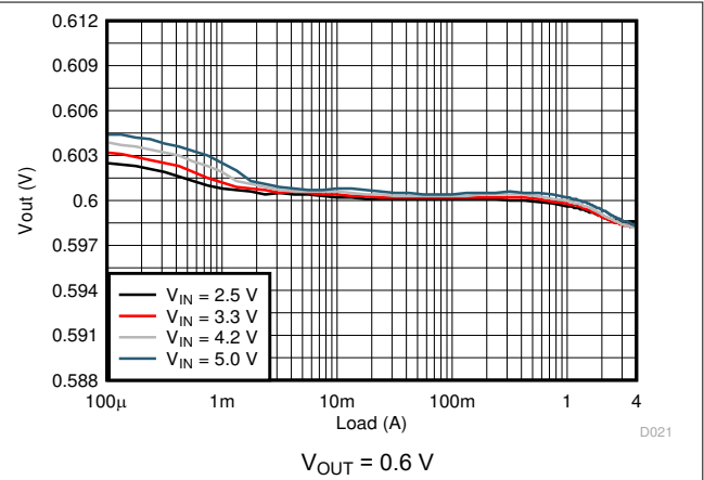
图 9-4. Load Regulation
