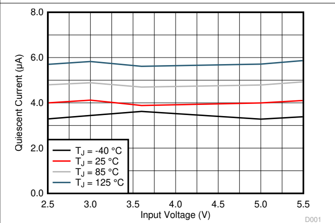
图 7-4. Quiescent Current
