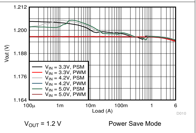
图 9-7. Load Regulation
