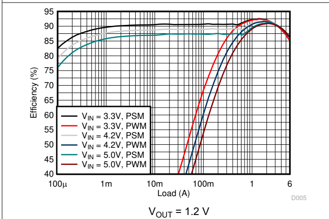
图 9-6. Efficiency
