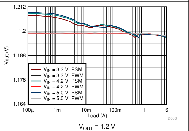
图 9-7. Load Regulation
