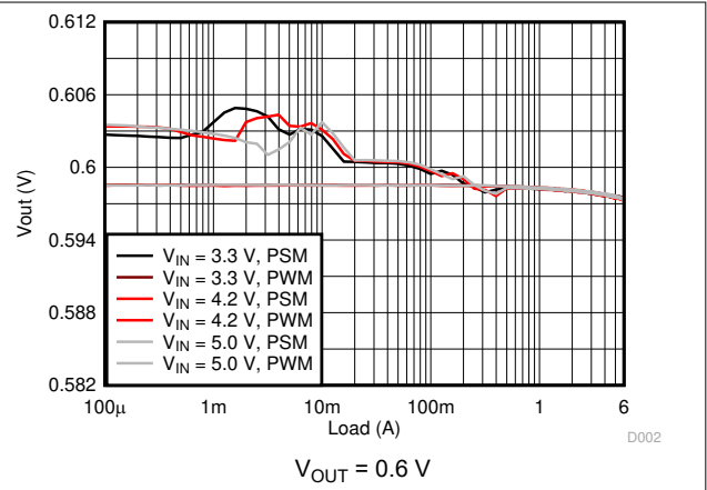
图 9-3. Load Regulation
