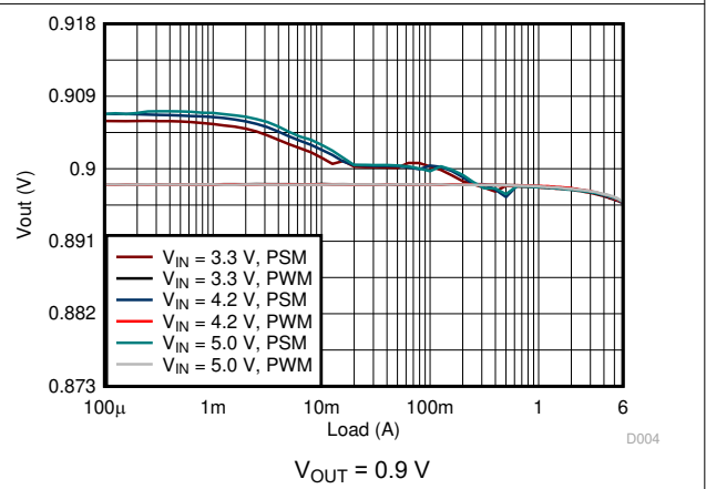
图 9-5. Load Regulation
