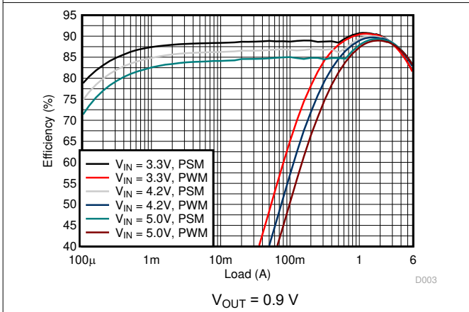
图 9-4. Efficiency
