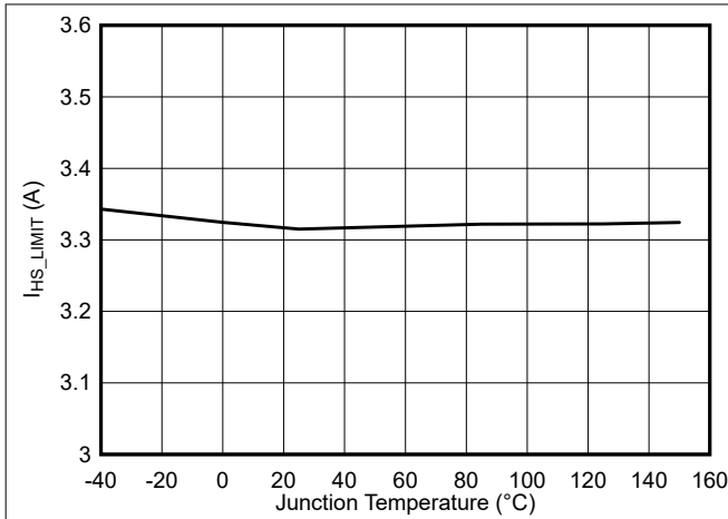
图 8-13. TPS62932 高侧电流限值与结温间的关系
