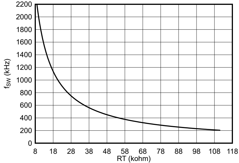
图 9-3. 开关频率与 R T 间的关系
