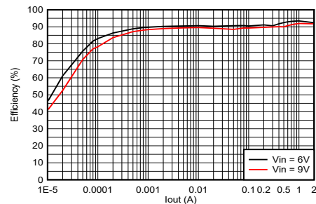
效率与输出电流间的关系 (3.3 V O , 2.5MHz, 1µH, 自动 PFM 或 PWM)
