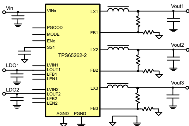
应用电路原理图
