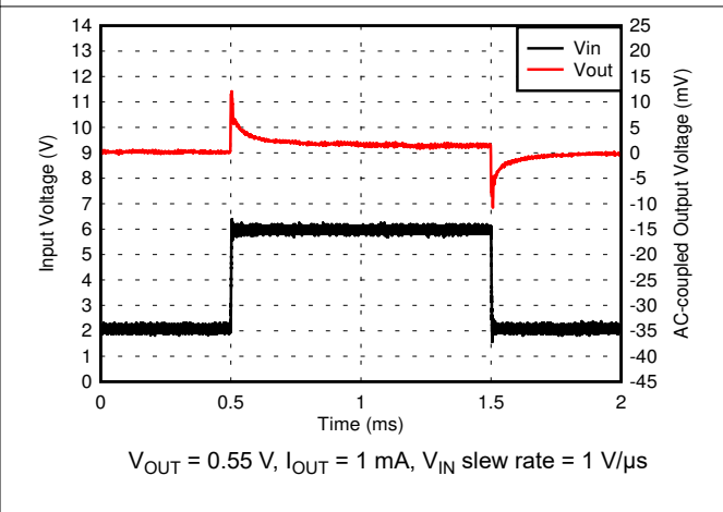
图 6-24. 0.55-V Line Transient
