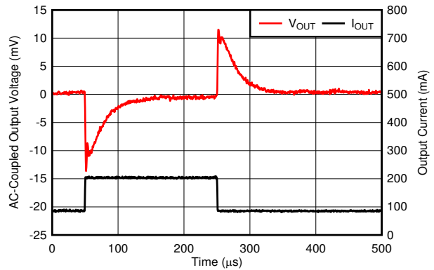
图 6-62. Load Transient
