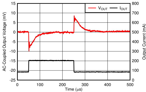
图 6-61. Load Transient
