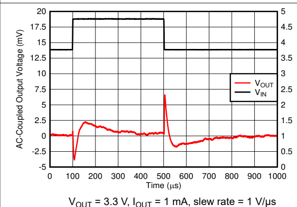
图 6-24. Line Transient
