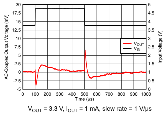
图 6-16. Line Transient
