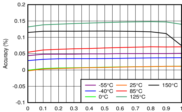
图 6-3. Output Accuracy vs V_{IN}
