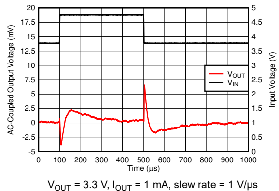
图 6-16. Line Transient
