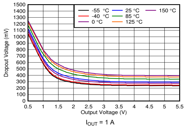
图 6-6. Dropout vs Output Voltage
