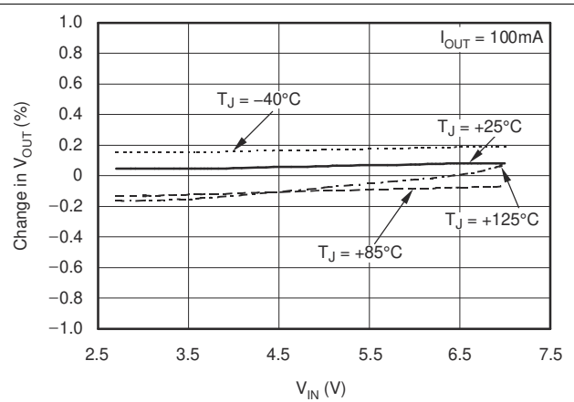
图 6-2. Line Regulation
