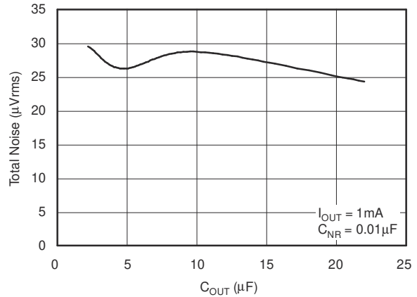
图 6-20. TPS799285 Total Noise vs C_{OUT}
