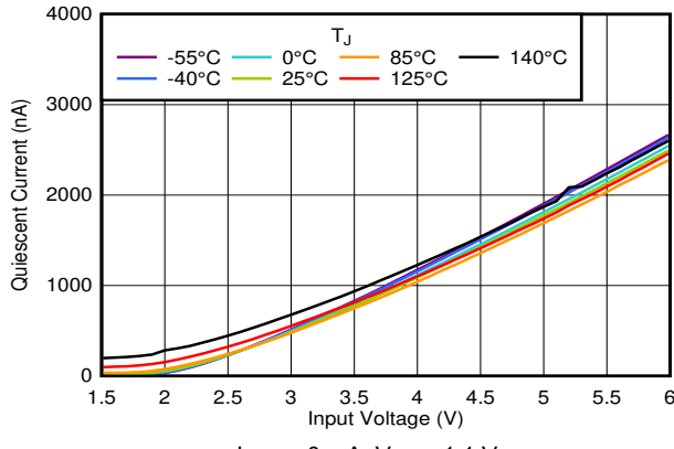
图 6-9. I_Q vs V_{IN} and Temperature
