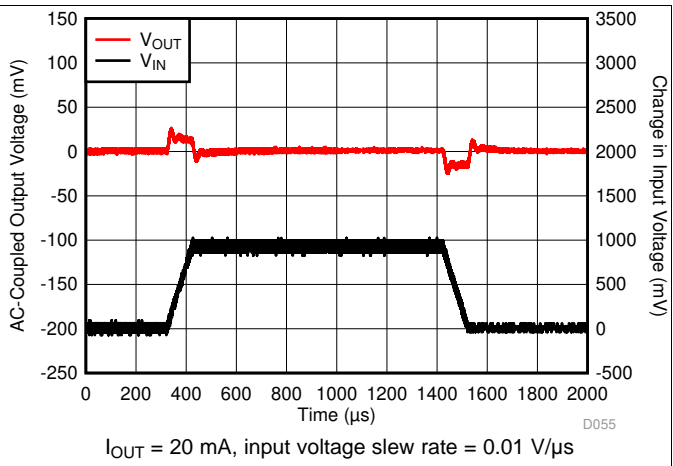
图 20. V_{IN} Transient
