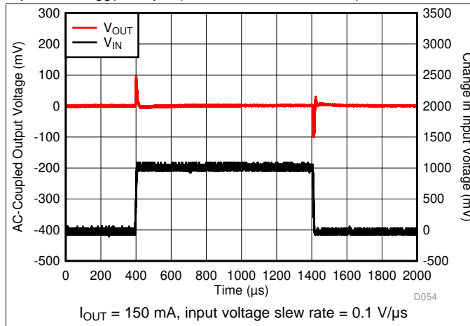
图 19. V_{IN} Transient
