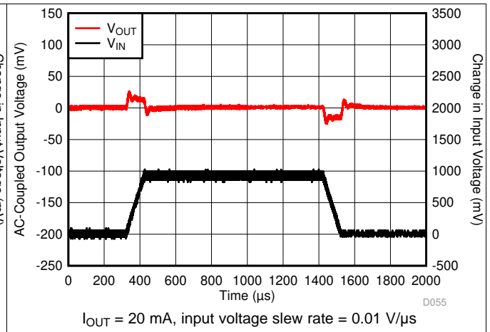
图 20. V_{IN} Transient
