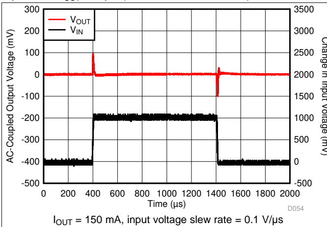
图 19. V_{IN} Transient
