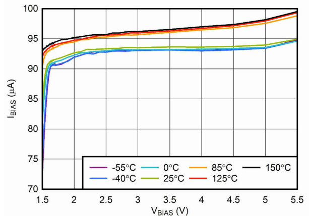
图 6-6. V_{BIAS} Input Current vs V_{BIAS}
