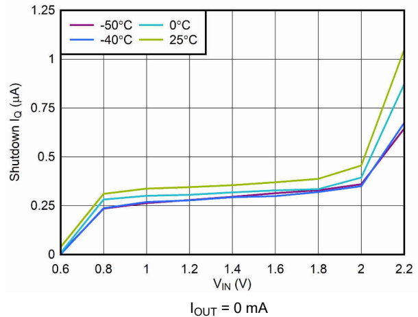
图 6-8. V_{\text{IN}} Shutdown I_{\text{Q}} vs V_{\text{IN}}
