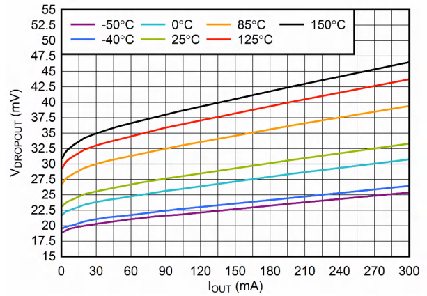
图 6-4. V_{IN} Dropout Voltage vs I_{OUT}
