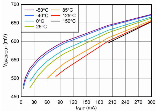
图 6-5. V_{BIAS} Dropout Voltage vs I_{OUT}
