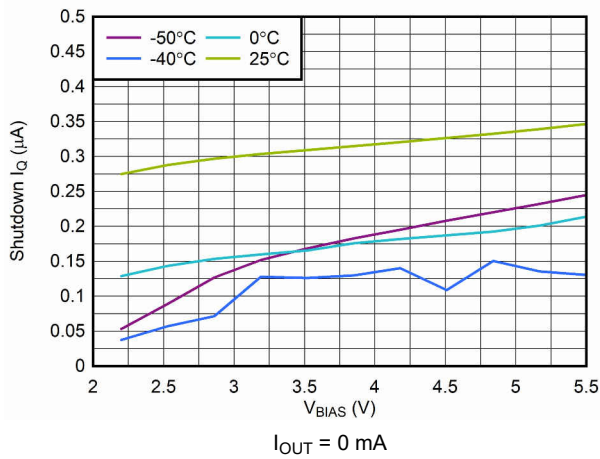
图 6-9. V_{\text{BIAS}} Shutdown I_{\text{Q}} vs V_{\text{BIAS}}
