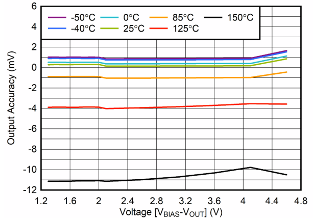
图 6-2. Output Voltage Accuracy vs V_{BIAS}
