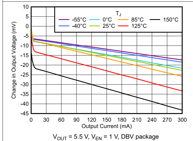
图 6-11. Load Regulation vs I_{OUT}
