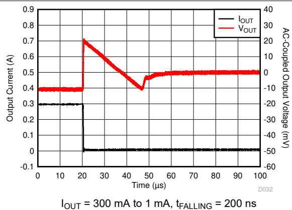
图 6-54. Load Transient
