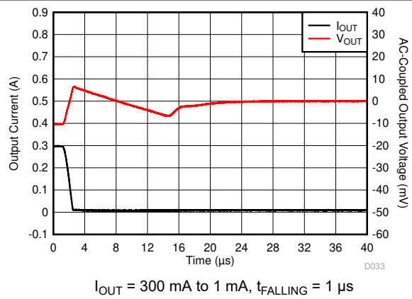
图 6-52. Load Transient
