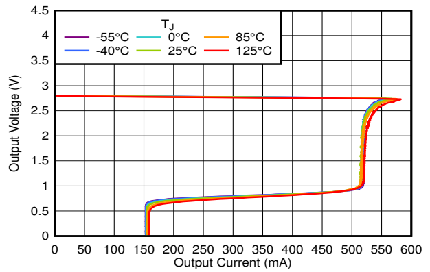
图 6-44. Current Limit
