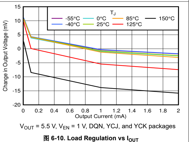
图 6-10. Load Regulation vs I_{OUT}
