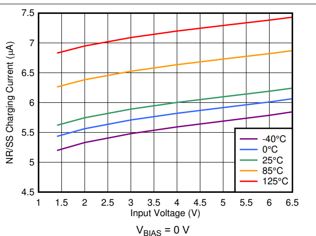
图 7-36. INR/SS Current vs Input Voltage
