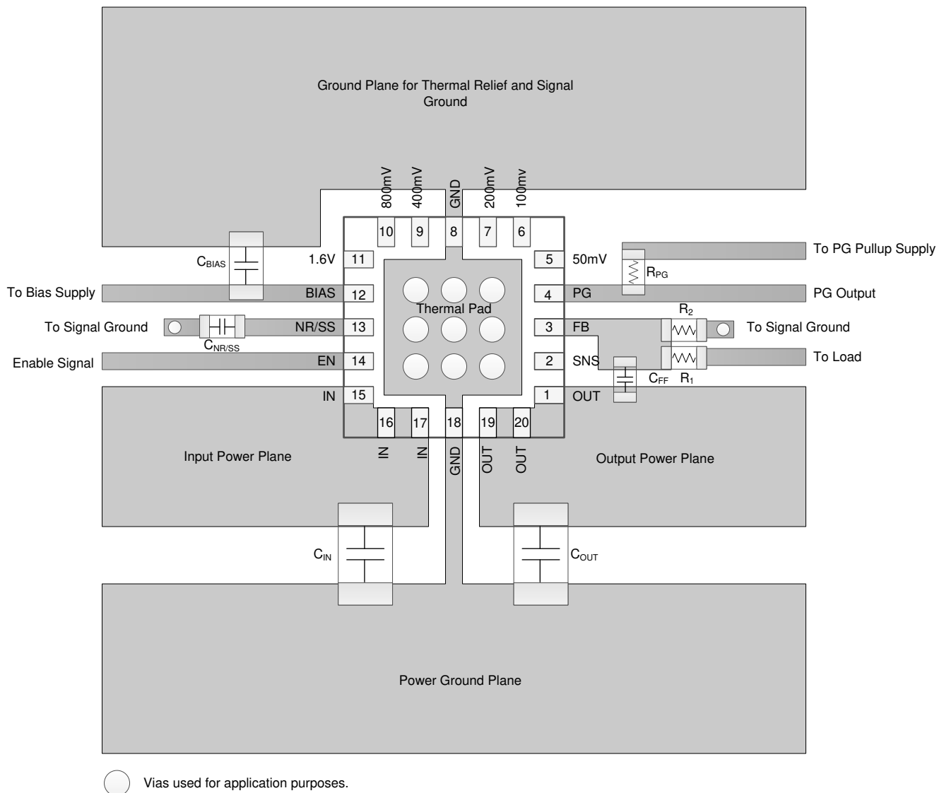
图 11-1. Example Layout
