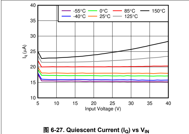
图 6-27. Quiescent Current ( I_Q ) vs V_{IN}
