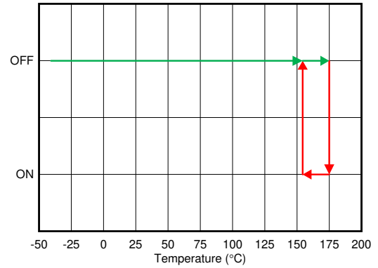
图 6-38. Thermal Shutdown
