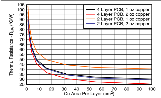
图 8-2. R_{\theta JA} vs Copper Area (DDA Package)
