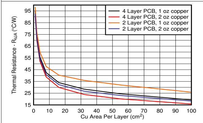
图 8-4. R_{\theta JA} vs Copper Area (KVU Package)
