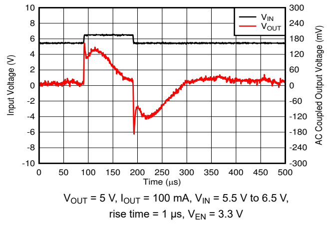
图 6-16. Line Transients
