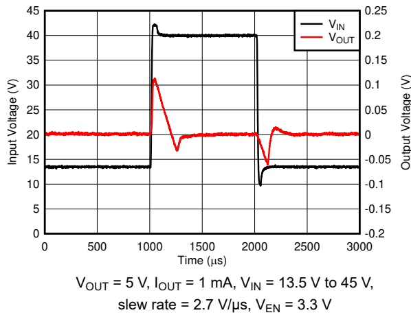
图 6-15. Line Transients
