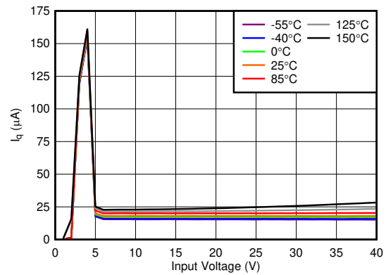
图 6-26. Quiescent Current ( I_Q ) vs V_{IN}
