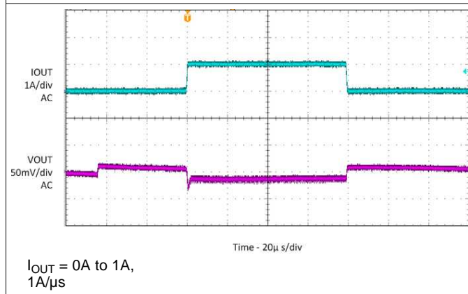
图 26. Load Transient
