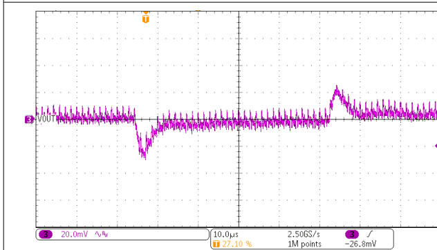
图 8-4. 10-A Transient Load Step
