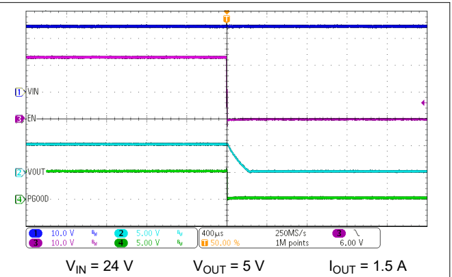
图 9-3. Enable Shutdown Waveforms
