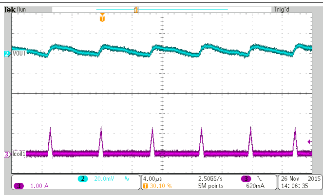
图 25. Output Discharge
