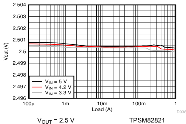
图 9-19. Load Regulation
