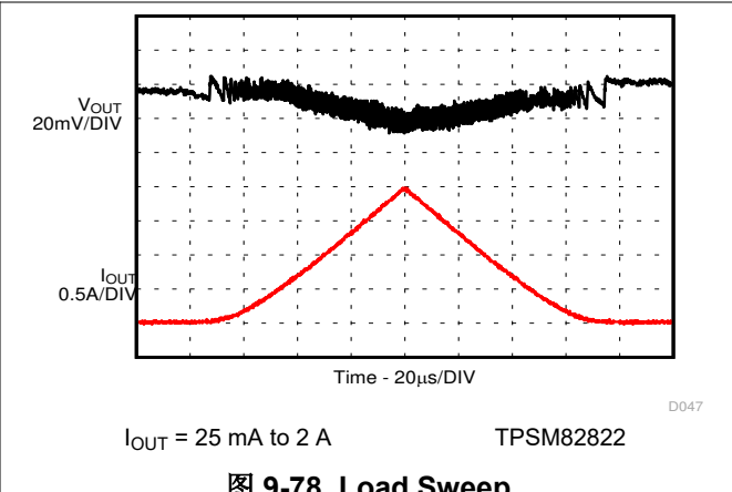
图 9-78. Load Sweep
