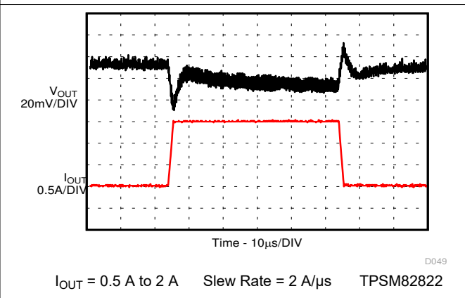
图 9-80. Load Transient
