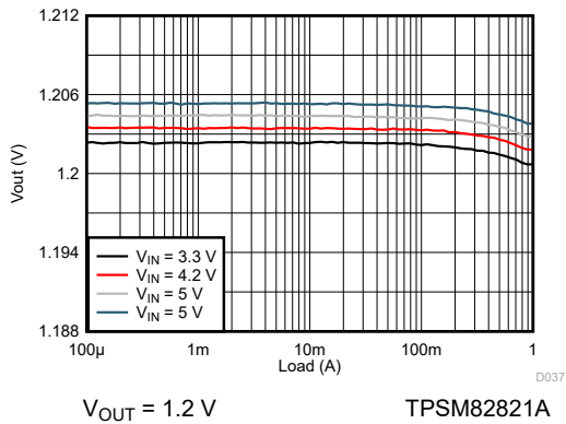
图 9-43. Load Regulation
