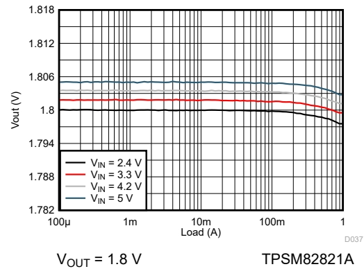
图 9-44. Load Regulation
