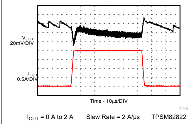
图 9-79. Load Transient
