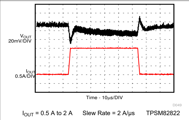
图 9-80. Load Transient
