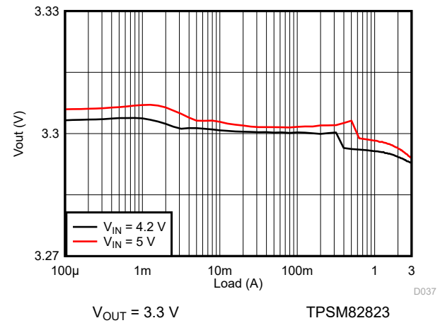
图 9-127. Load Regulation
