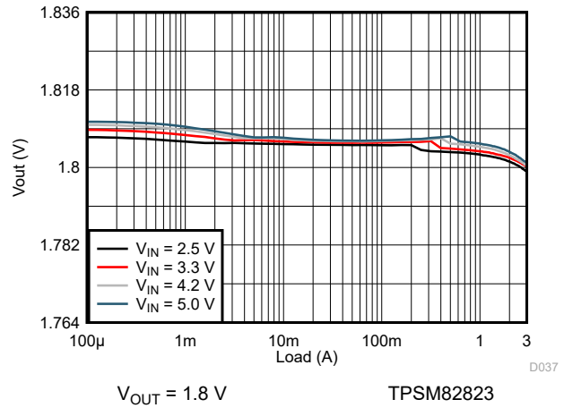
图 9-125. Load Regulation
