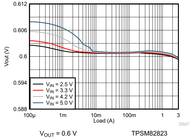
图 9-123. Load Regulation
