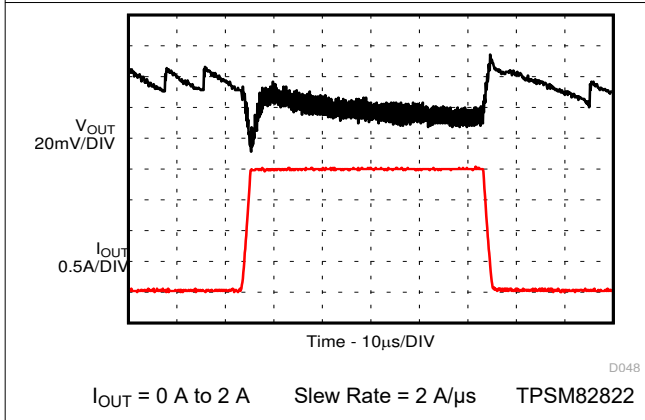
图 9-79. Load Transient
