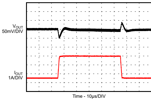
图 9-130. Load Sweep
