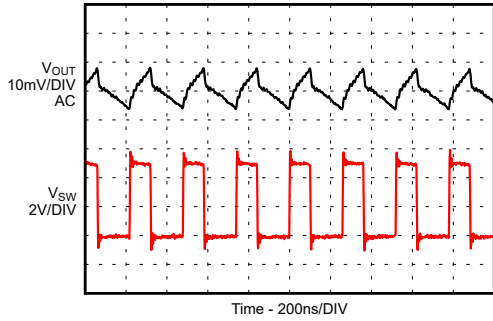
图 9-128. Output Ripple in PWM Mode
