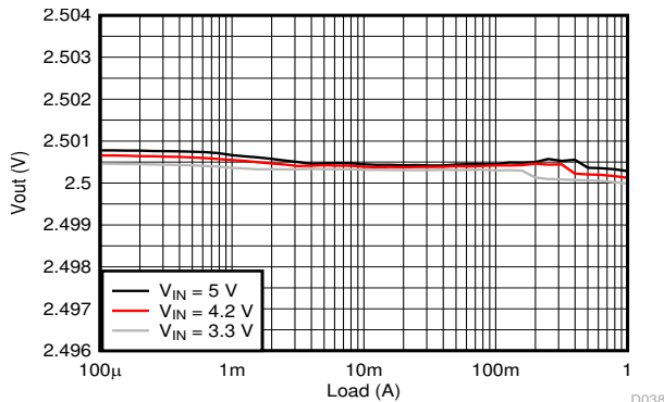
图 9-19. Load Regulation
