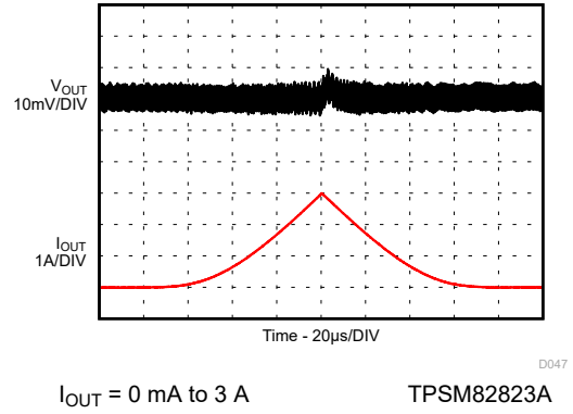
图 9-156. Load Sweep
