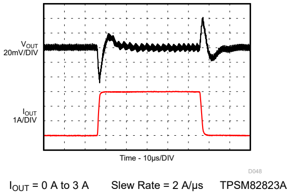
图 9-157. Load Transient
