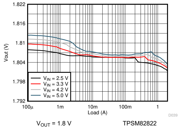
图 9-68. Load Regulation
