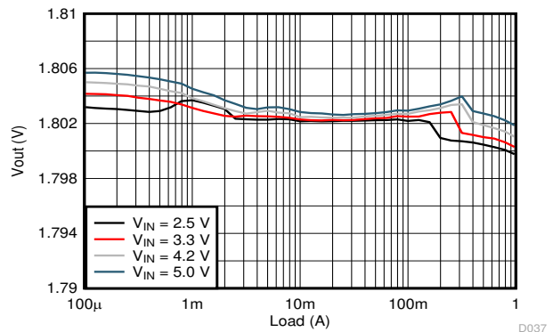
图 9-18. Load Regulation
