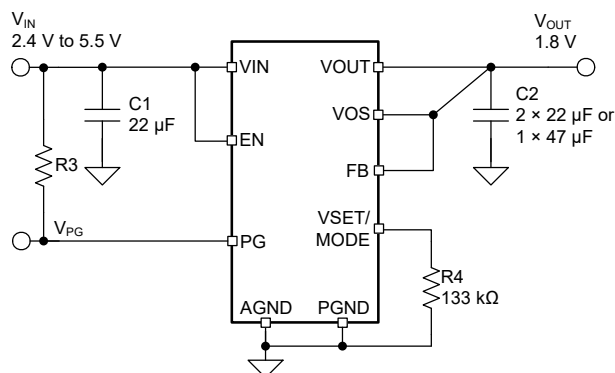
典型应用原理图 - 固定输出电压选项
