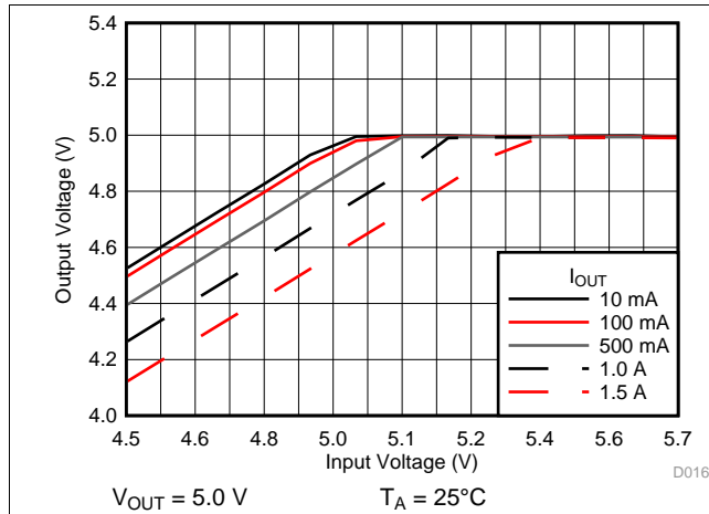
图 16. Drop-Out Voltage
