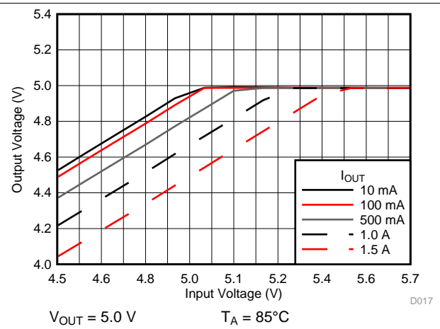
图 17. Drop-Out Voltage
