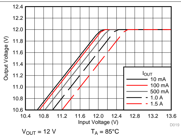
图 19. Drop-Out Voltage
