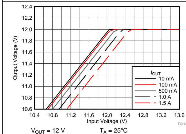
图 18. Drop-Out Voltage
