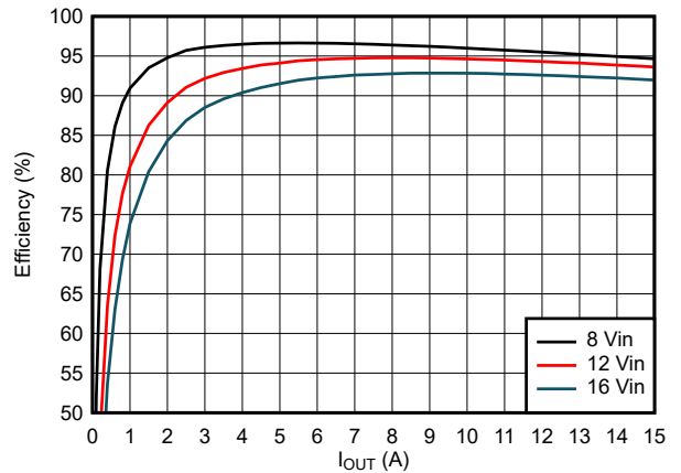
图 8-7. Efficiency
