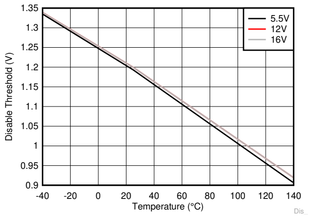
图 6-11. Disable Threshold
