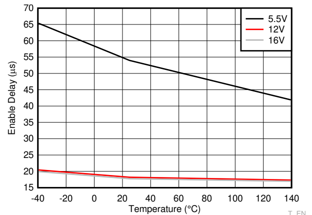
图 6-12. Enable Delay
