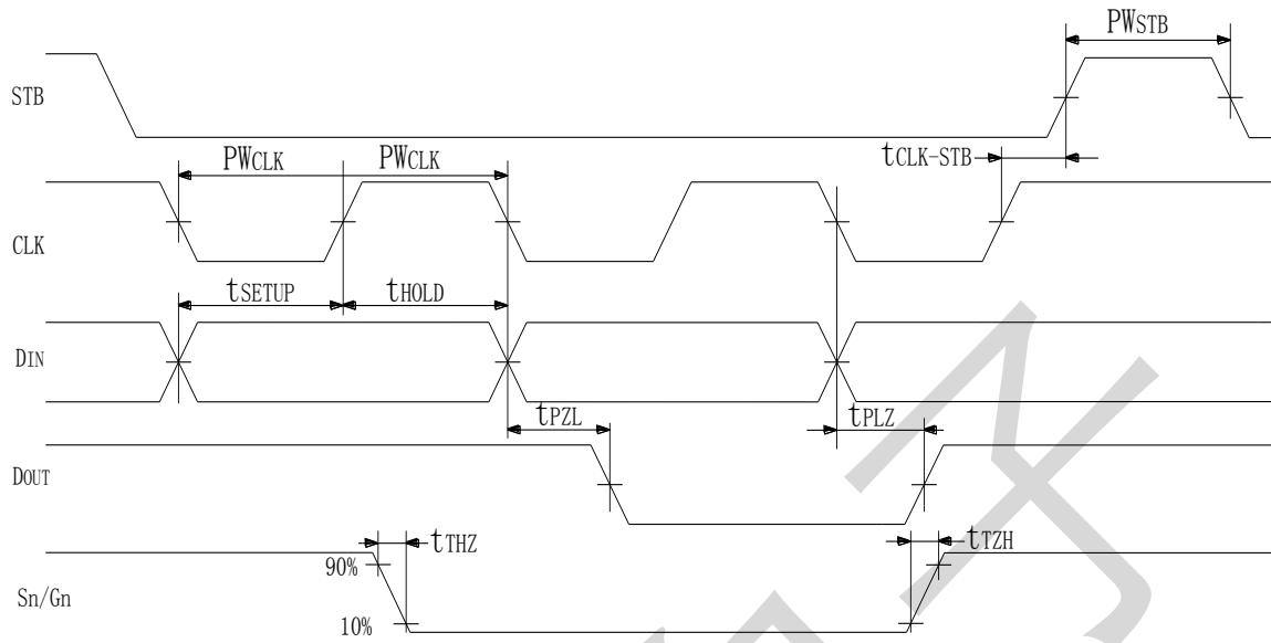
时序波形图
